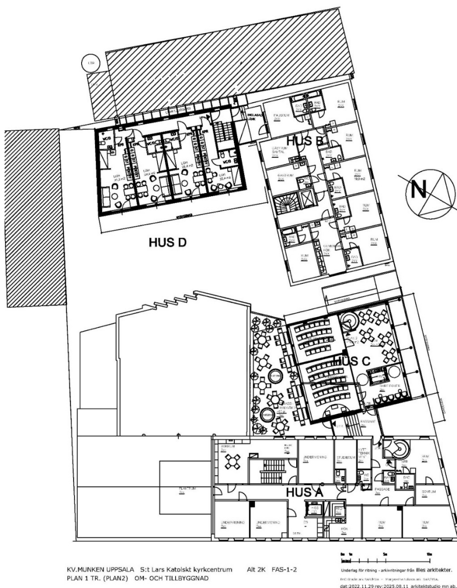
Figur 21 Illustrationsplan, första våningen. Befintlig kyrka markeras som hus A, tillbyggnad som ska fungera som ny entré och mötesrum markeras som hus C, systrarnas hus markeras som hus B, nya lokaler och gästlägenheter på gården markeras som hus D. Källa: Arkitektstudio MN.
