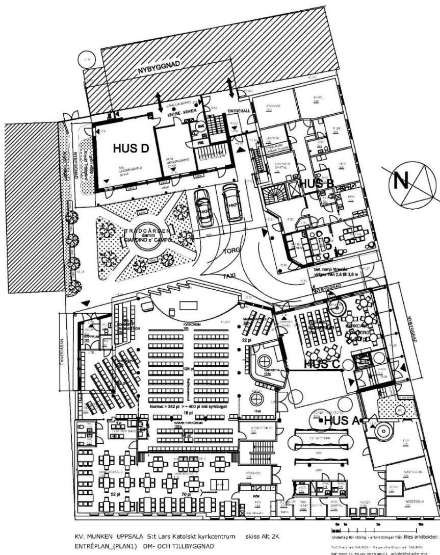
Figur 20 Illustrationsplan, bottenvåning. Befintlig kyrka markeras som hus A, tillbyggnad till kyrkobyggnaden markeras som "nybyggnad", tillbyggnad som ska fungera som ny entré och mötesrum markeras som hus C, systrarnas hus markeras som hus B, nya lokaler och gästlägenheter på gården markeras som hus D. Källa: Arkitektstudio MN.
