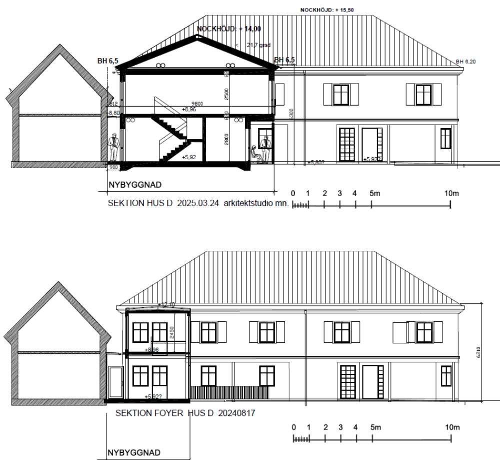
Figur 22 Sektioner genom nya huset D och intilliggande huset på Grillska gården. Källa: Arkitektstudio MN.
