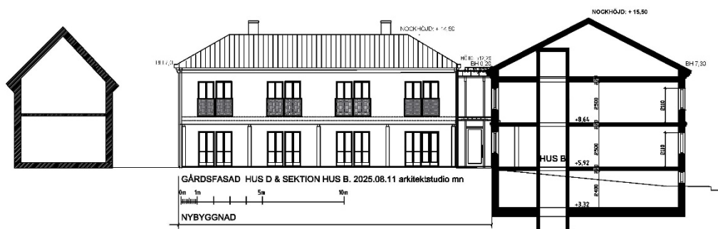
Figur 25 Sektion genom systrarnas hus och hus på grannfastigheten Fjärdingen 30:5 med fasad av nya hus D mot gården. Vy från innergården mot hus D. Källa: Arkitektstudio MN.
