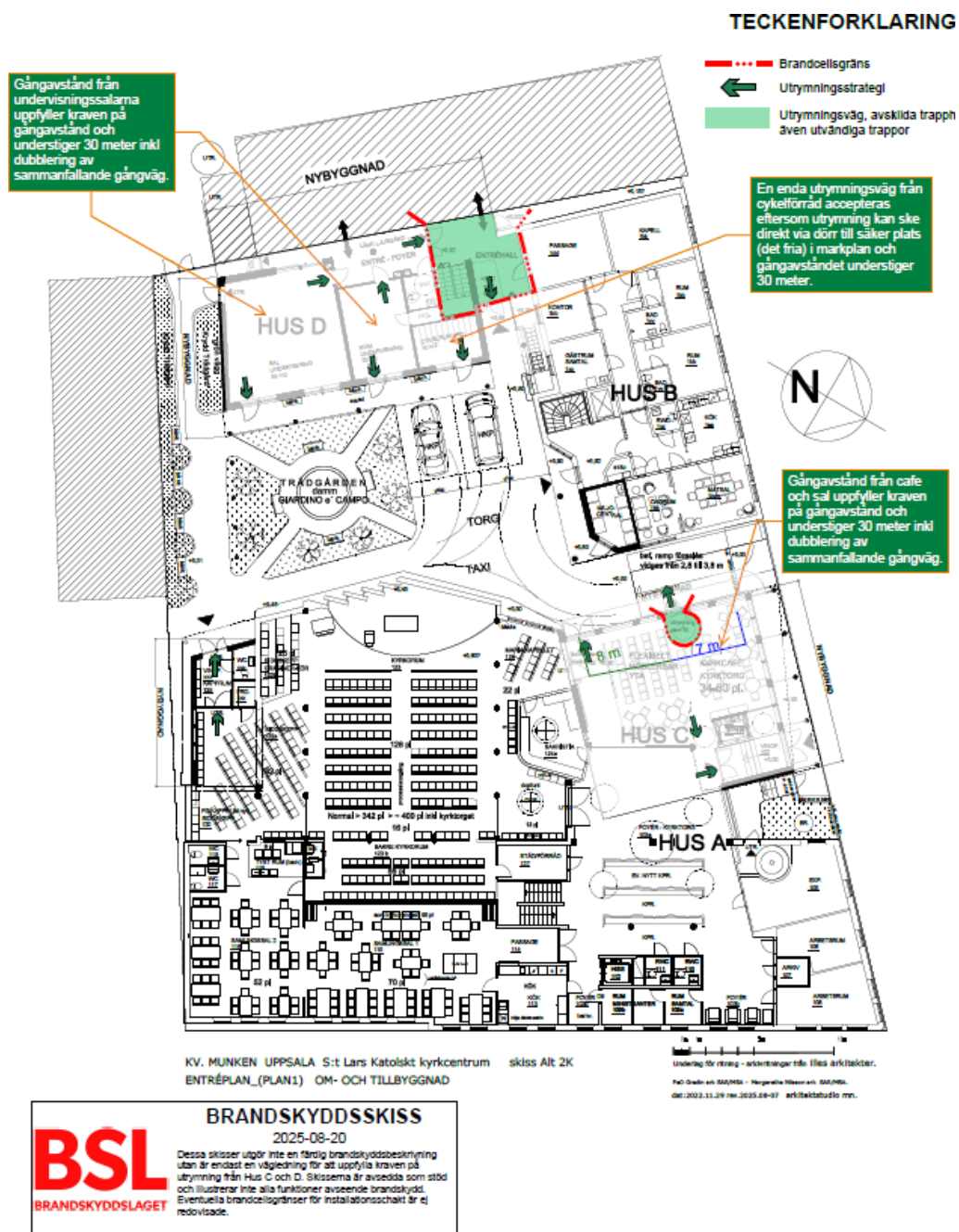
Figur 58 Illustrationsplan som visar utrymningsvägar i bottenvåning. Källa: BSL brandskyddslaget.
