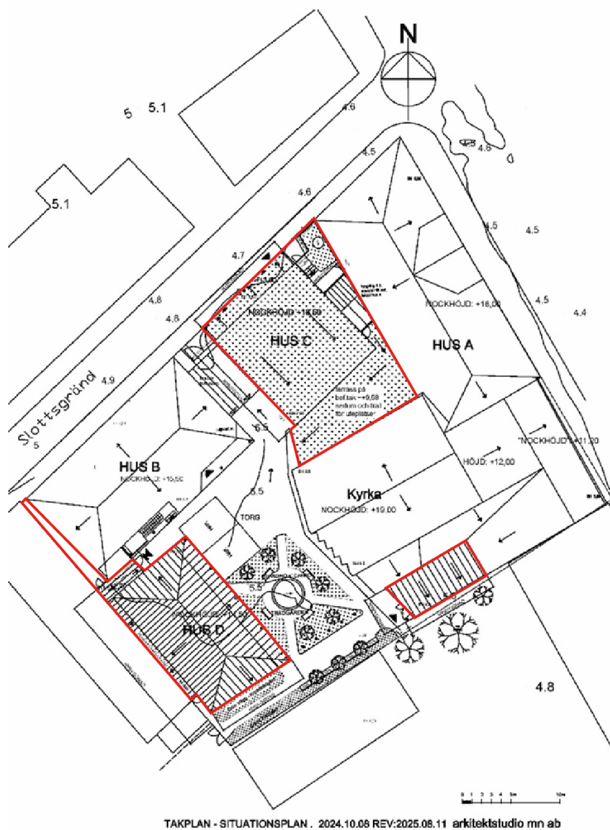
Figur 16 Situationsplan. Ny bebyggelse - hus C, hus D och tillbyggnad till kyrksalen, markerade med röd avgränsning. Källa: Arkitektstudio MN.
