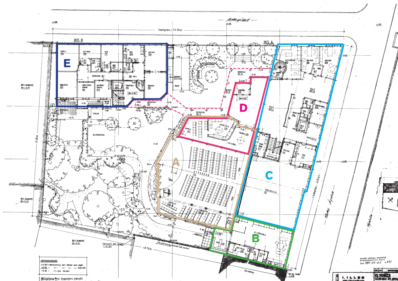
Planritning för bottenplan som även visar utemiljöns utformning samt hur byggnadsvolymer samspelar med utemiljön och varandra. På planritningen framgår även de olika volymerna som utgör delar av den sammantagna kyrkobyggnaden.
