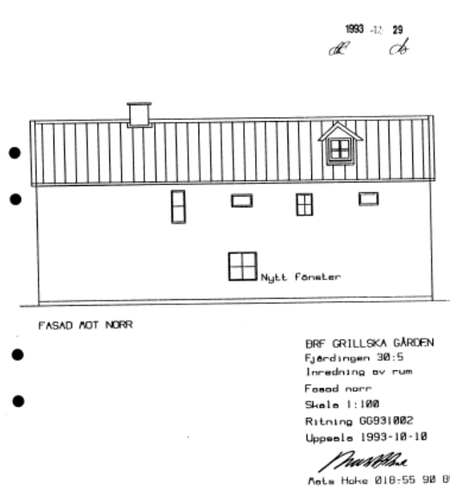
Figur 6 utdrag från bygglovshandlingar för Trädgårdsgatan 16F och G, fasadritning. Fönster som täcks av skuggan vid solnedgång kl. 18 den 21 juni markeras som "Nytt fönster" i bygglovshandlingar från 1993.
