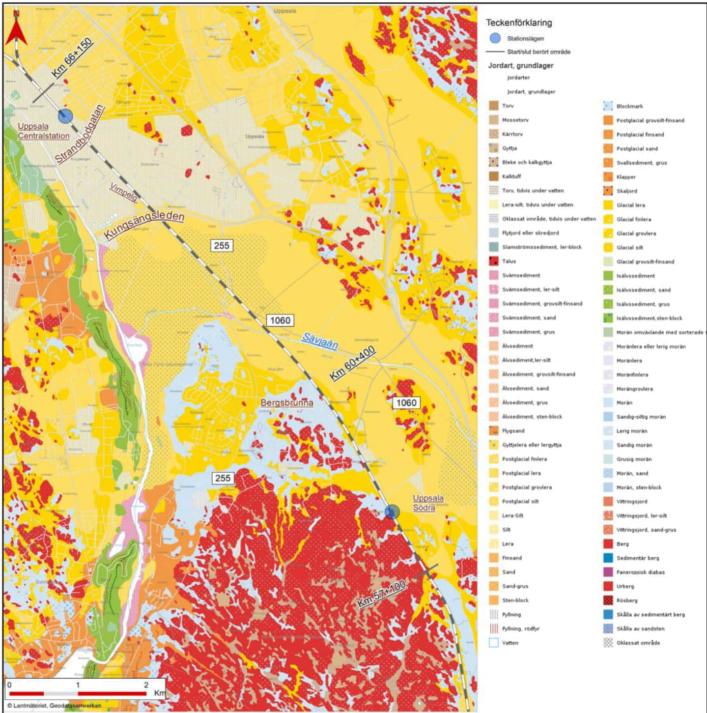
Figur 5. Jordartskarta.
