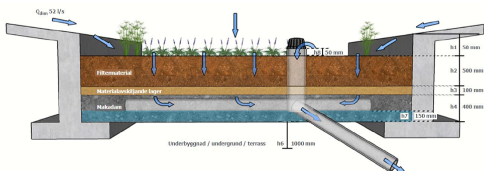
Figur 36 Förslag på uppbyggnad av regnväxtbädd med tät botten för omhändertagande av dagvatten från trafikerade ytor
