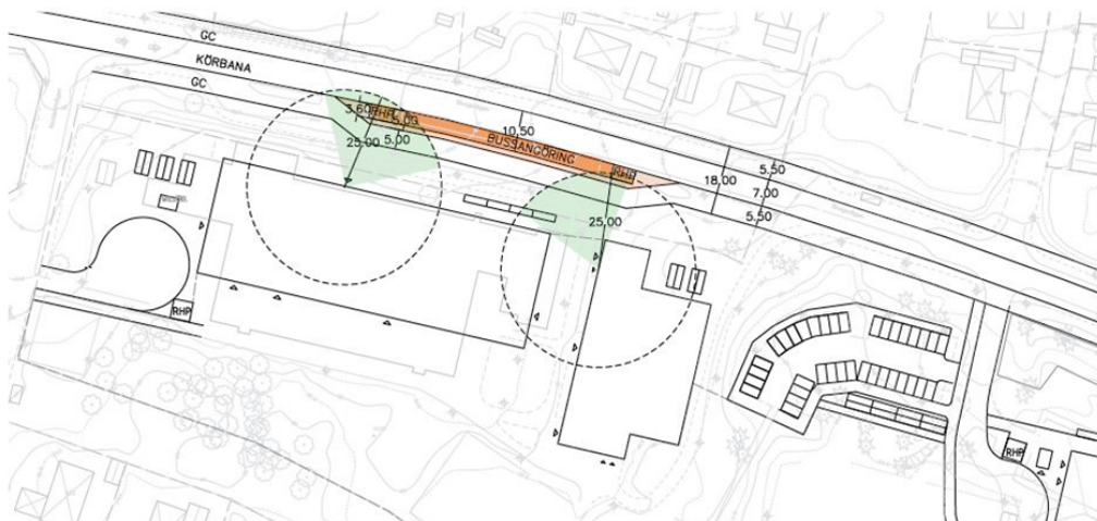
Figur 32 Angöringslösning till Uppsävjaskolan anpassad efter gatusektion enligt intentioner i den fördjupande översiktsplanen för de sydöstra stadsdelarna. Orange yta markerar en flexyta avsedd för färdtjänst, buss och parkering för rörelsehindrade (besökare).
