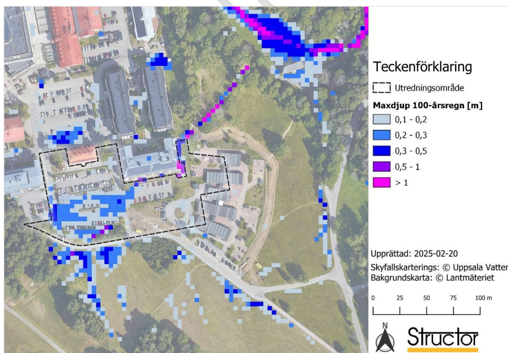
Bild 58. Flygbild där maximalt djup vid ett 100-årsregn är markerat. Det som planläggs som kvartersmark inom planområdet är markerat med en svart, streckad linje. Den privata förskola som ligger nedströms planområdet är markerad med en röd ellips. Observera att den temporära förskolan som syns i planområdets östra del är nedmonterad. Illustration: Structor (2025)
